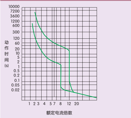
图11 NM1-1250动作特性曲线
