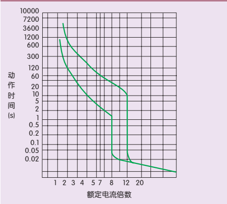
图9 NM1-630、800动作特性曲线
