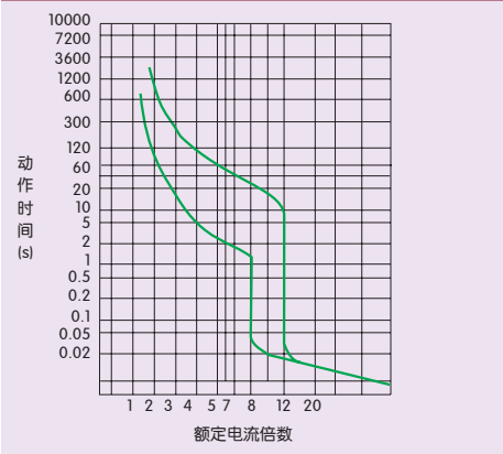
图7 NM1-400动作特性曲线
