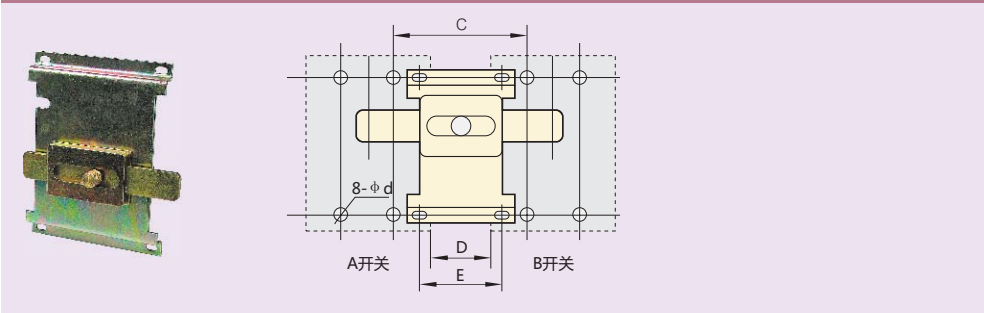
安装尺寸图(见表14)
